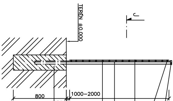
ŘEZ J-J
